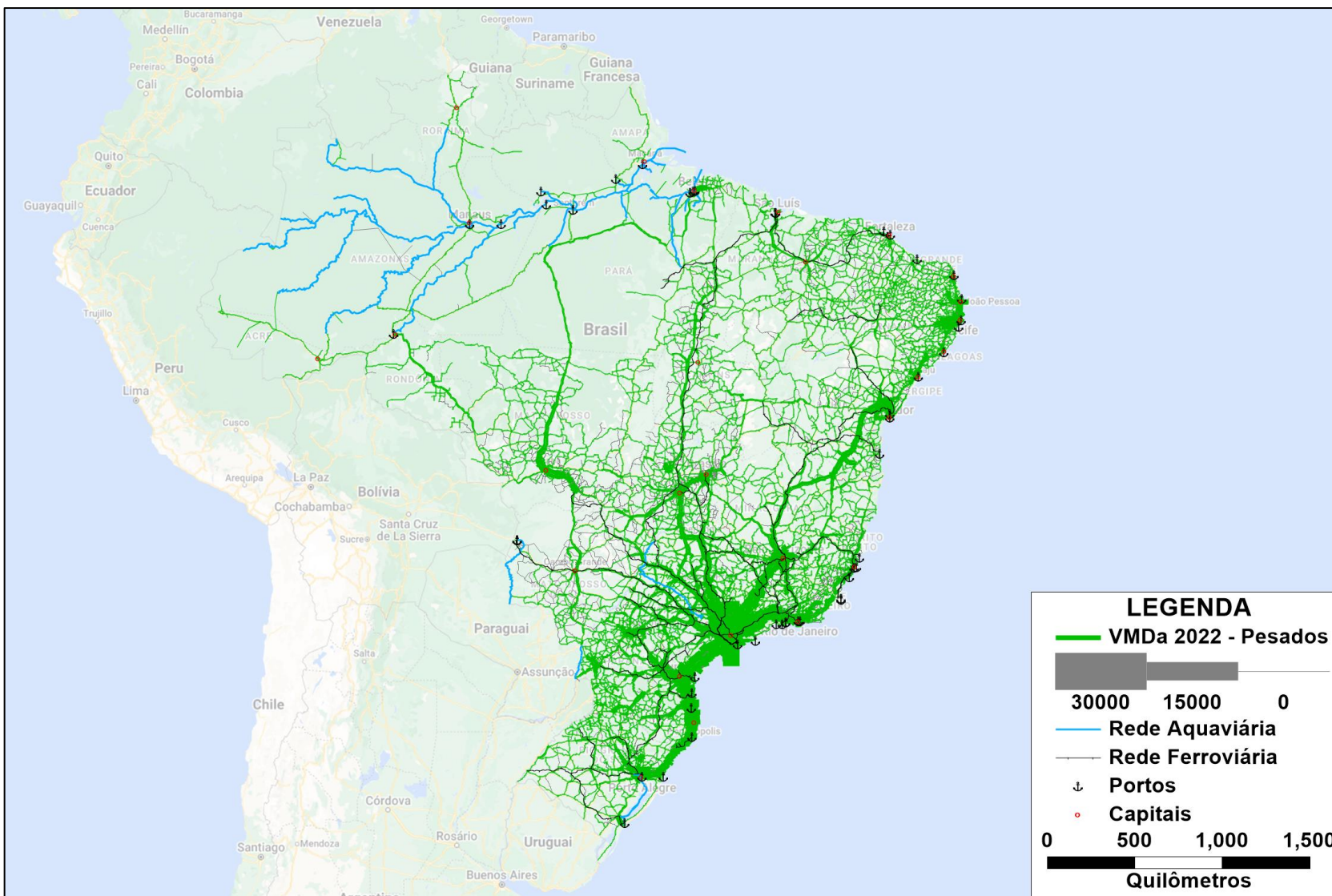
Figura 6.4 – Resultados da Alocação de Fluxo de Veículos Pesados em rede para o Cenário 22
