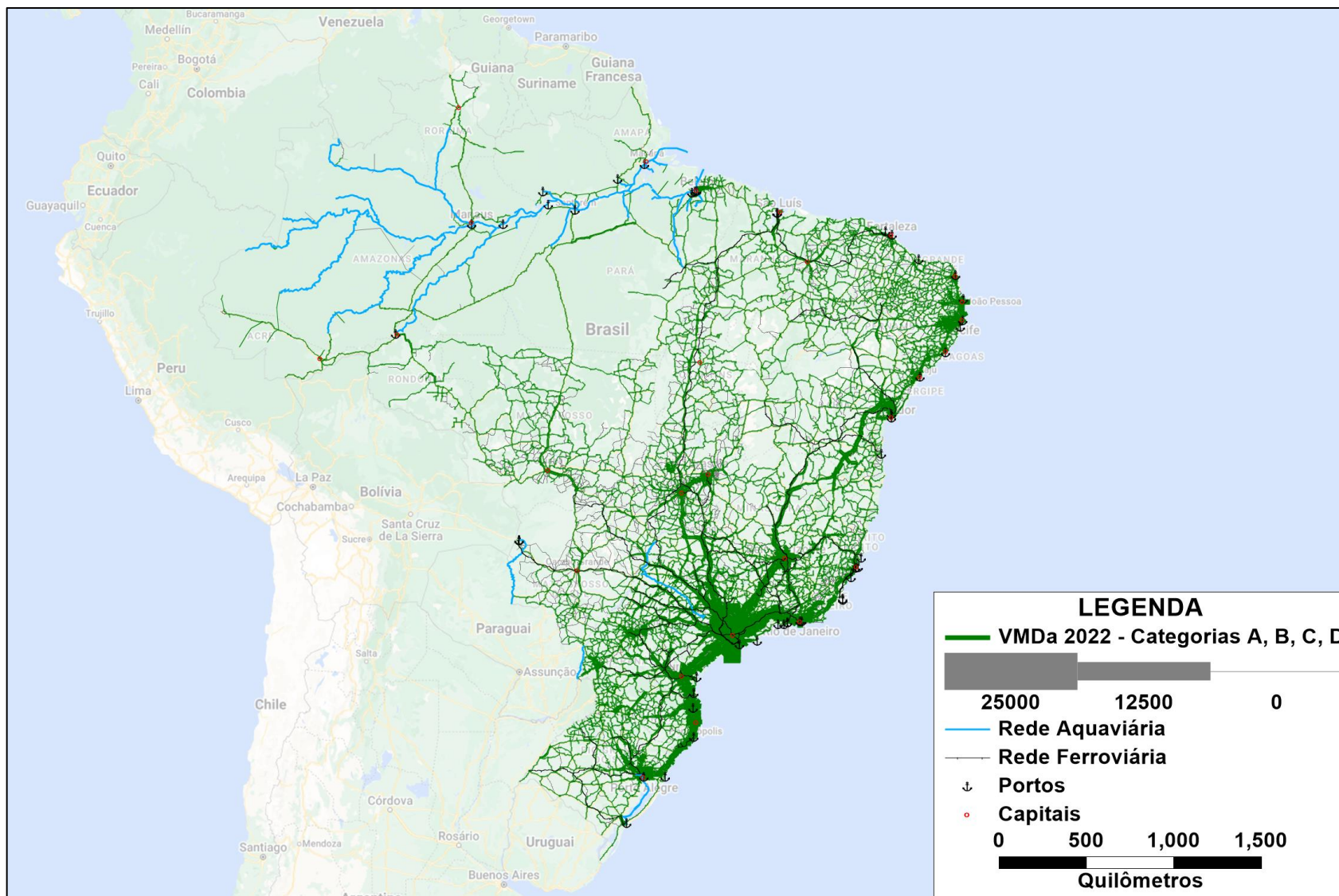
Figura 6.5 – Resultados da Alocação de Fluxo de Veículos Pesados (Categorias A, B, C e D) em rede para o Cenário 22
